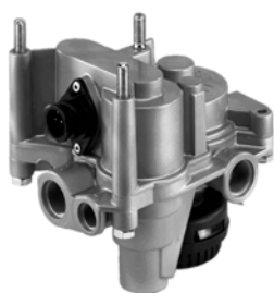
Рис. 19: Пропорциональный ускорительный клапан
