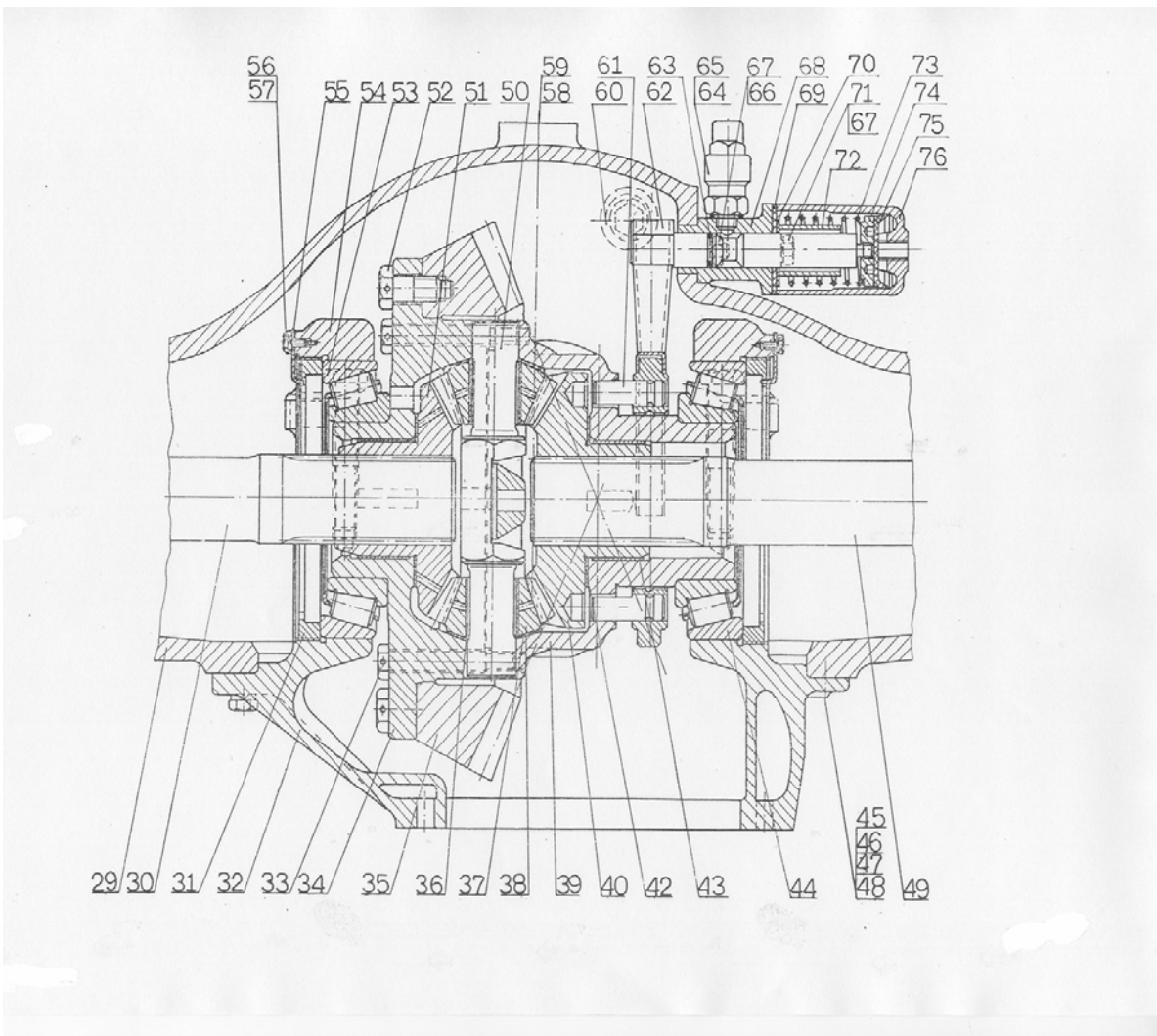
Рис.2. Дифференциал
