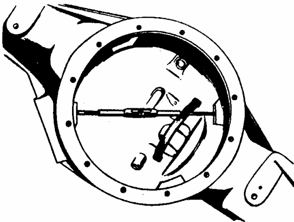
Рис.14. Замер диаметра \Phi 340H8
