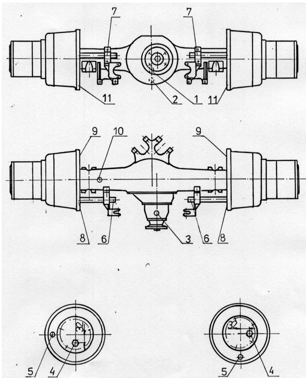
Рис.22. Места пробки и пресс-масленки
