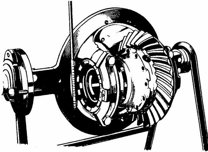
Рис.6. Ключ Т 17 - 393 для опорного кольца подшипника дифференциала
