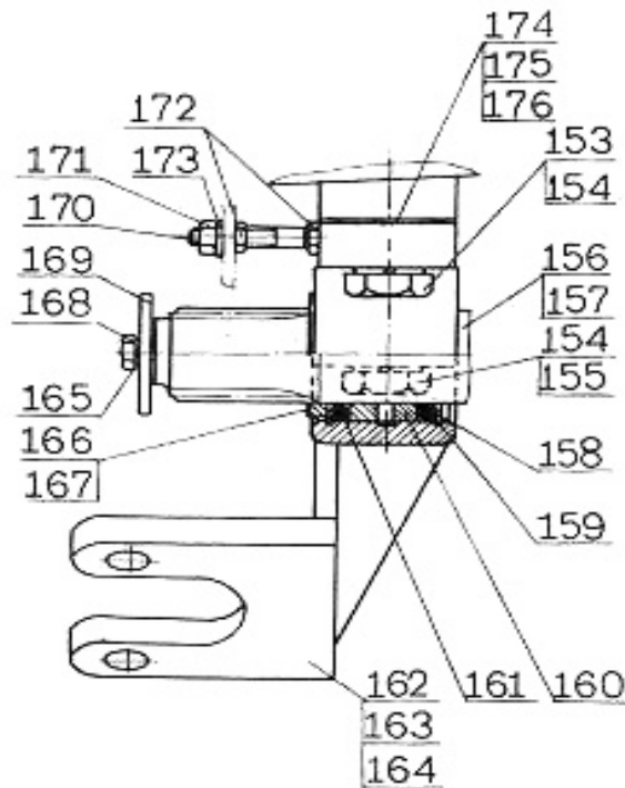
Рис.4. Рычаги разжимных кулаков
