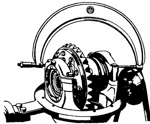
Рис.15. Замер скобой размера 340 m7
