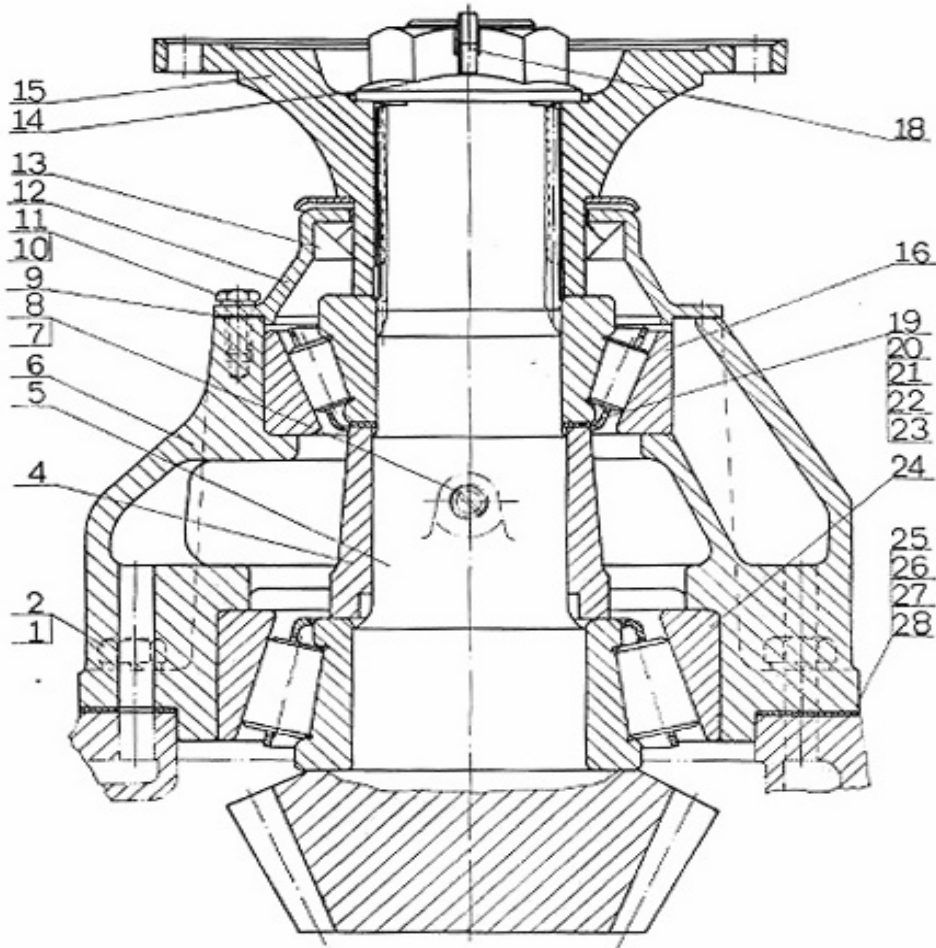
Рис.1. Ведущая шестерня главной передачи
