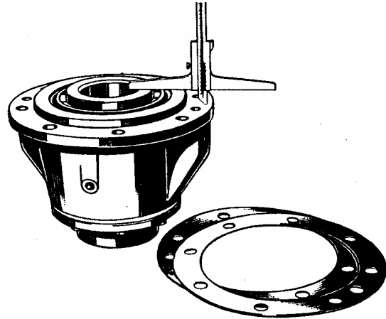
Рис.10. Замер расстояния О в стакане подшипников
