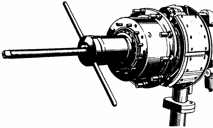
Рис.19. Набивание внутреннего кольца наружного подшипника
