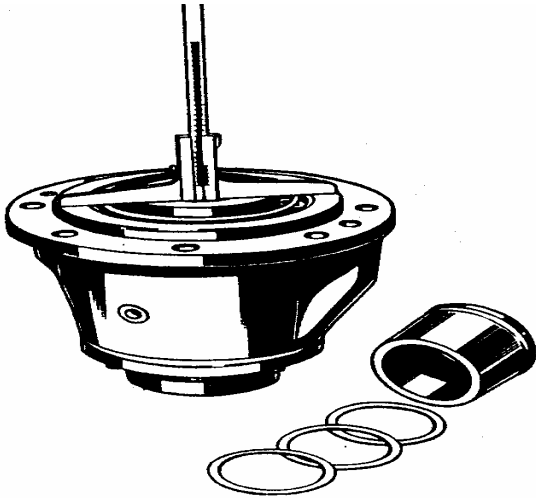
Рис.9. Замер расстояния Т в стакане подшипников
