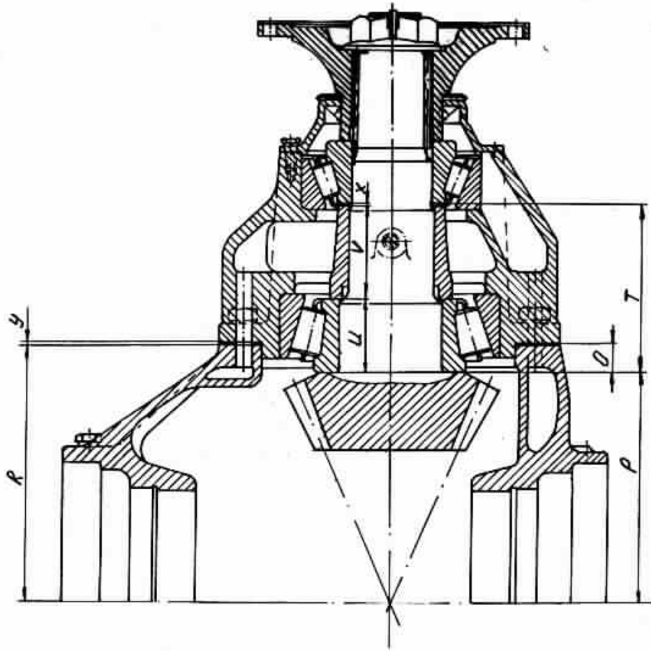
Рис.8. Расчет толщины регулировочных прокладок главной передачи
