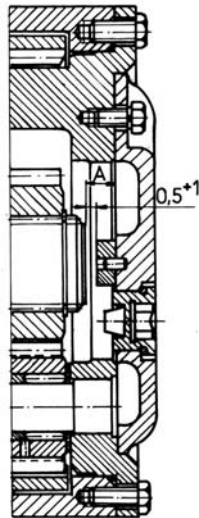
Рис.21. Замер расстояния А
