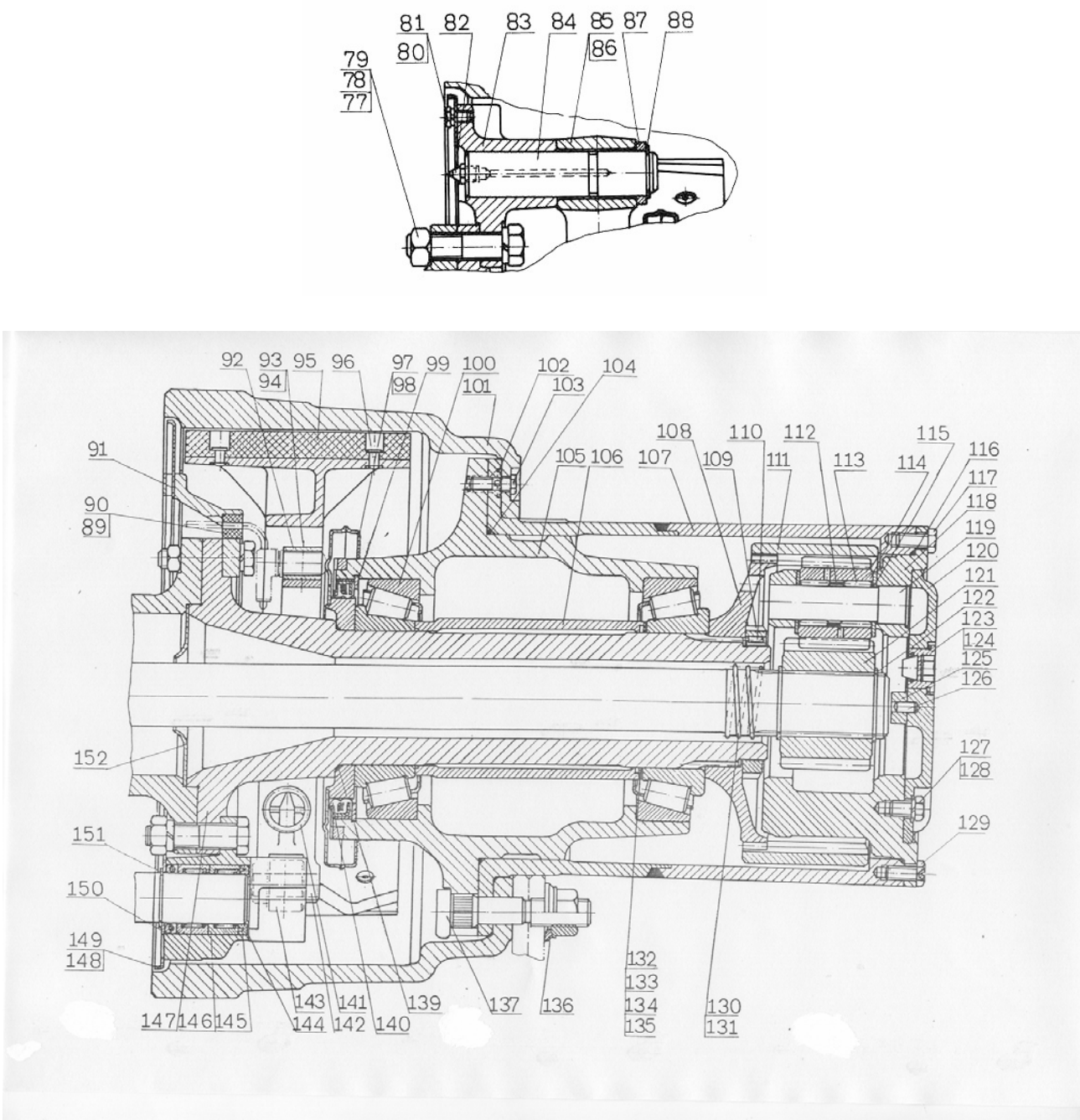
Рис.3. Тормозной механизм и колесный редуктор
