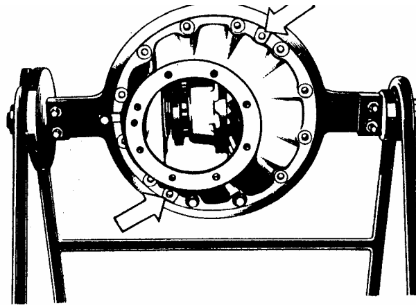
Рис.5. Отделительные болты для снятия картера главной передачи с заднего моста 397.2
